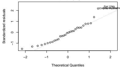
Normal Q-Q
